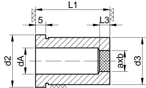
Tipo HKDF
